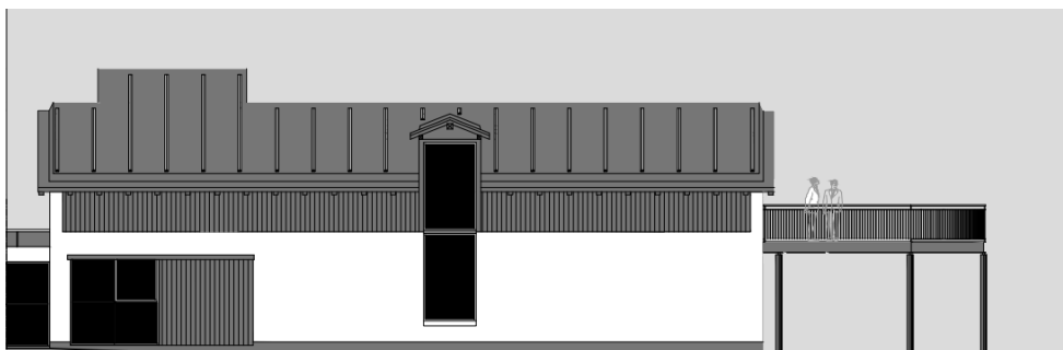
Ansøgte udformning af terrassen – under: eksisterende forhold
