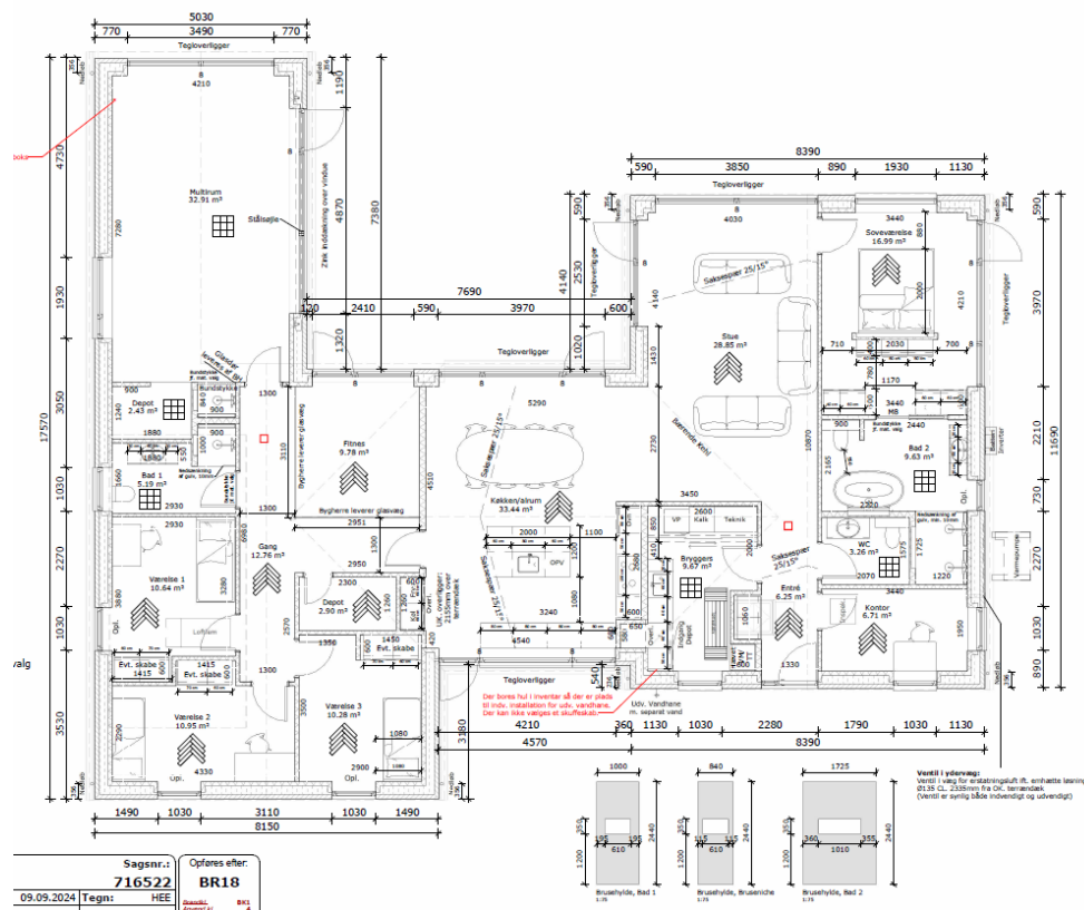
Grundplan bolig
