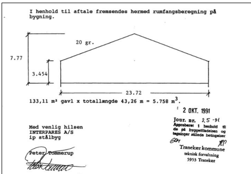
Fig. 4. Tilsendt af ansøger. Byggetegning af maskinhallen.
