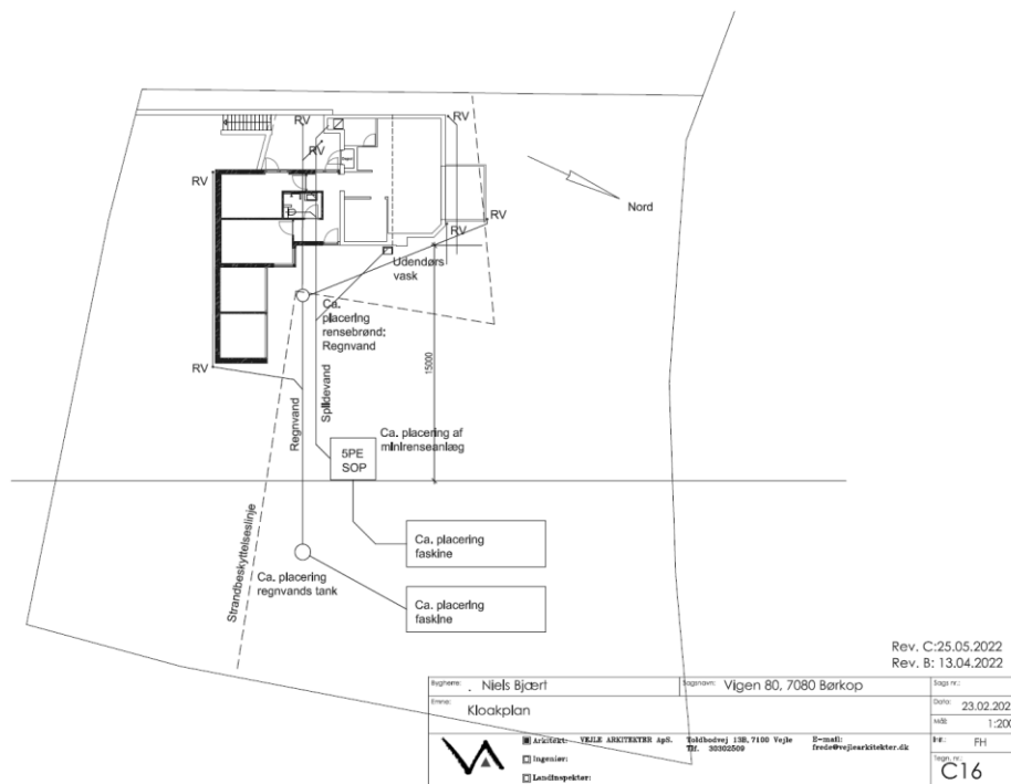
Fig. 2. Kloaktegning fra ansøgningen med angivelse af dækslernes placering.
