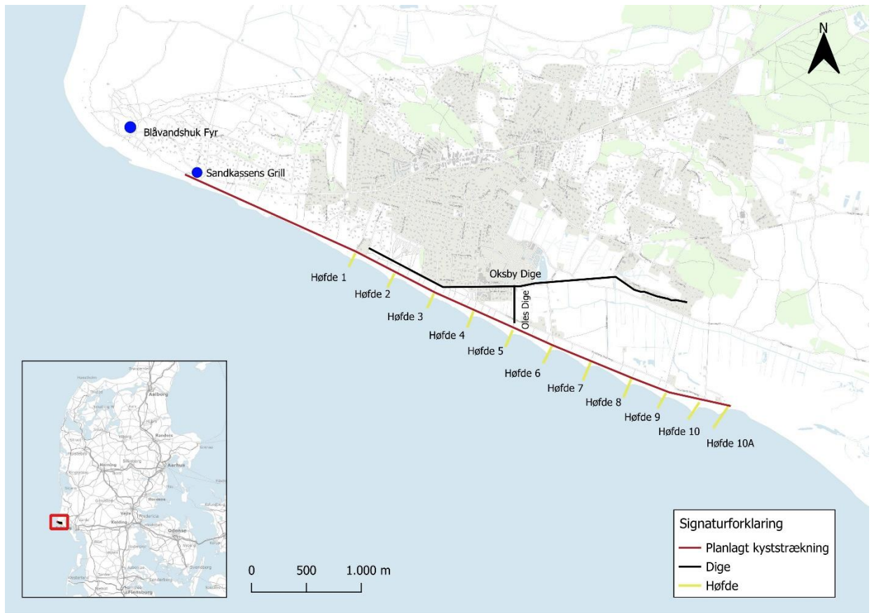
Figur 4-1. Eksisterende kystbeskyttelse og planlagt kyststrækning ved Blåvand. Det skal bemærkes, at selv om det ikke fremgår af figuren, findes der et stendige mellem høfde 1-6.
