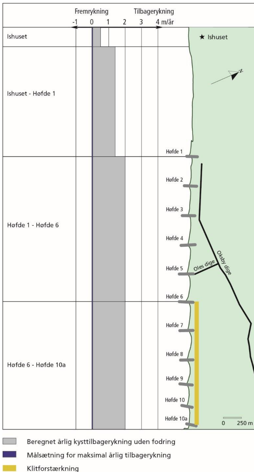
Figur 4-2. Målsætningen for maksimal kysttilbagerykning i perioden 2020-2024. Den naturlige tilbagerykning under eksisterende forhold er vist med grå skraver.
