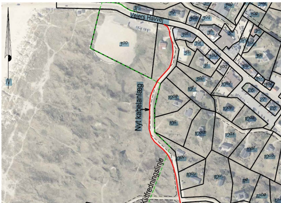
Fig. 2 Principskizze af den del jordkabeltrace, der ligger på klitfredet areal. Kabeltrace vises med rød linje. Grøn stiptet linje viser klitfredningslinjen (fra ansøgningen)
