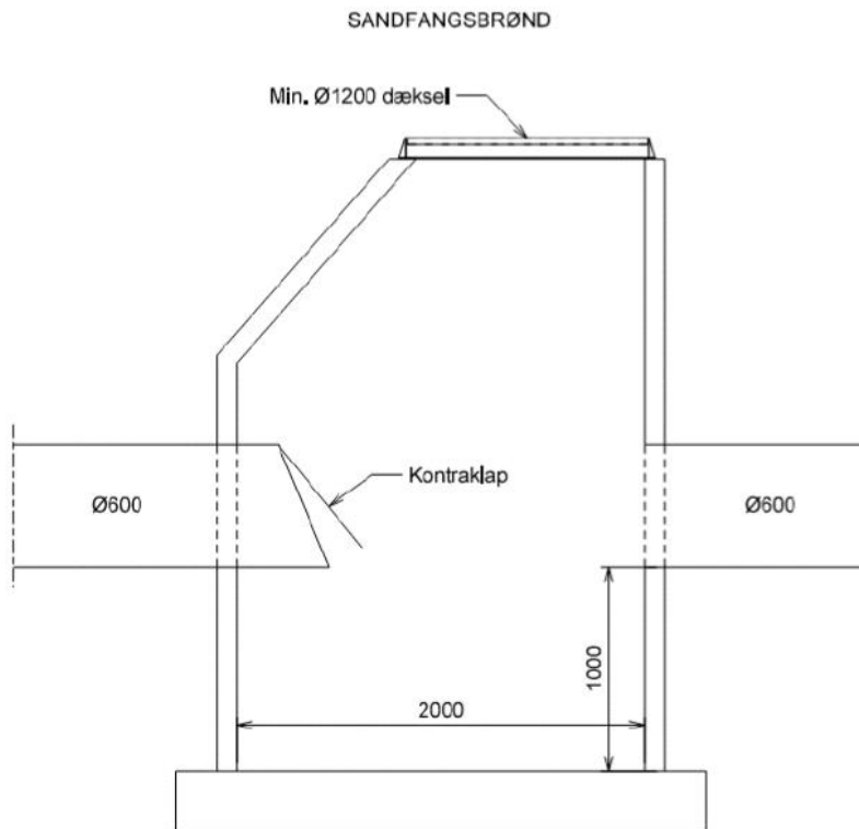
Fig. 8. Principskitse af sandfangs-brønd med kontraklap, indsendt af ansøger.
