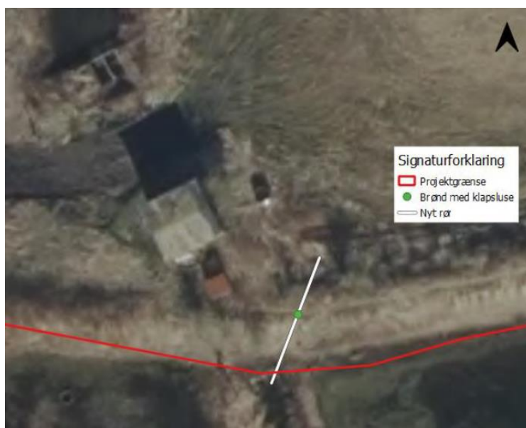
Fig. 7. Placering af rørforbindelse (hvid linje) mellem projektområdet og fjorden, indsendt af ansøger. Brøndens placering er markeret med en grøn cirkel.
