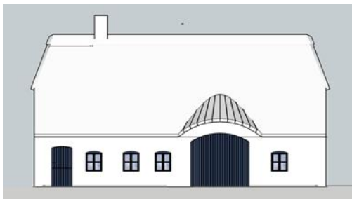
Øst (mod gårdsplads): 1 Vindue i nordlig del. Glasparti bag ved port.
