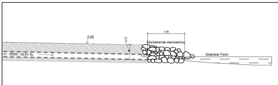
Detalje af snittegning af udløbet viser, at ledningen stopper før stensætningen og således ikke vil være synlig. Denne del forudsætter således ikke dispensation fra strandbeskyttelseslinjen.
