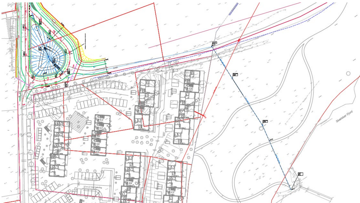
Tegning af projektet. Tegningen viser, at der er to brønde inden for strandbeskyttelseslinjen.
