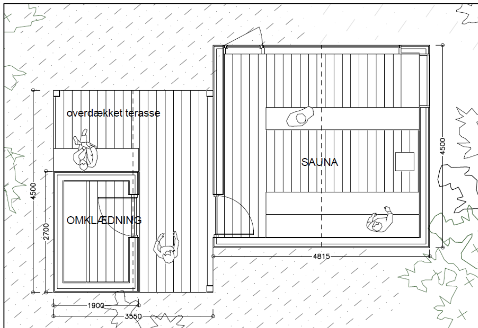
Grundplan for sauna med omklædningsfaciliteter. Saunaen er ca. 22. kvm og omklædningsfaciliteter er ca. 16 kvm inklusive terrasseareal.
