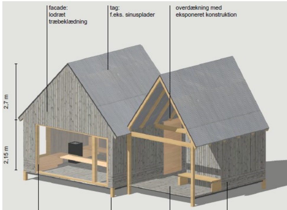
Visualisering af sauna med omklædningsfaciliteter. Den maksimale højde på bygningerne er 4,85 meter målt fra gulvplan. Bygningerne er hævet en anelse over jorden.
