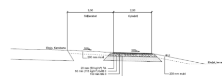
Snit G-G
