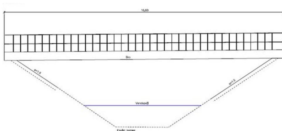
Fig.3. Snittegning af cykelsti-bro over Kastbjerg Å (fra ansøgningen)
