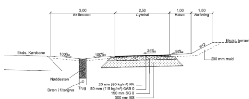
Snit D-D
