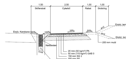
Snit E-E
