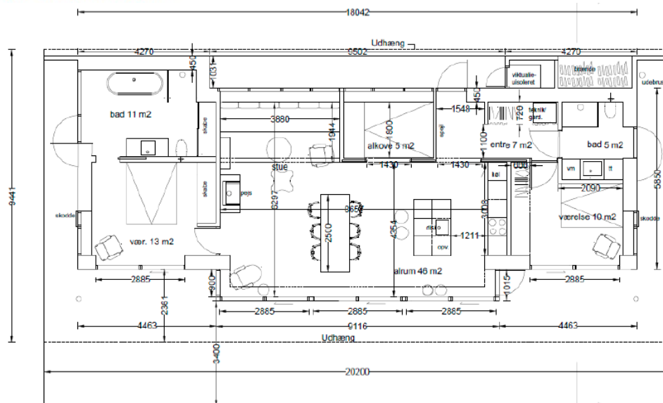
Figur 4: Grundplan for det fremtidige sommerhus
