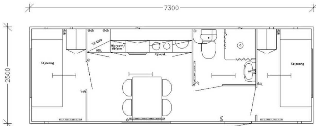
Fig. 4. Plantegning over eventvogn til 2 personer.
