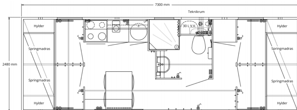
Fig. 6. Plantegning over eventvogn til 4 personer.
