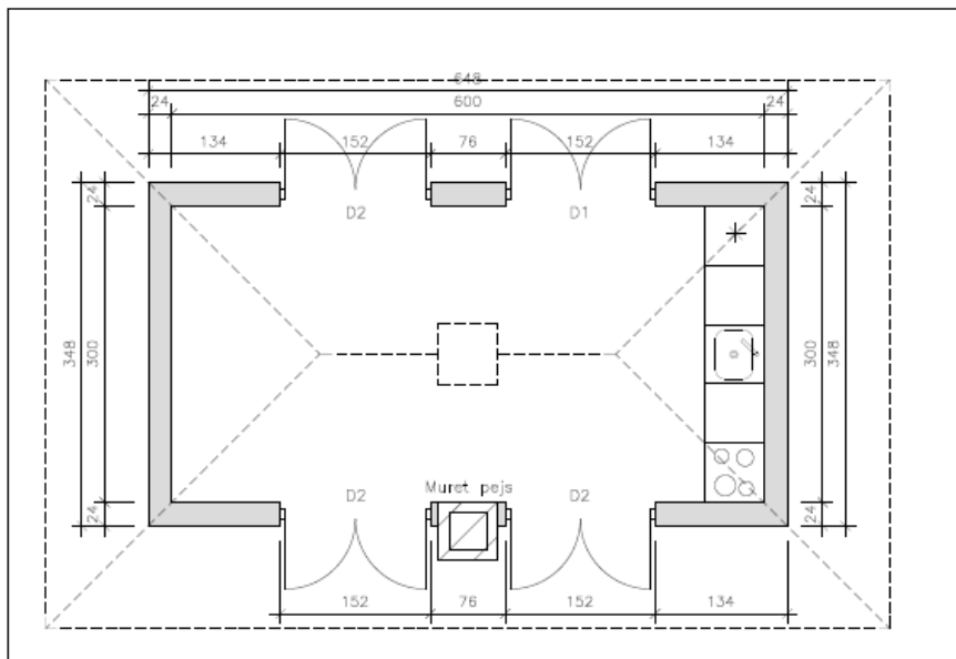
Grundplan ny bebyggelse
