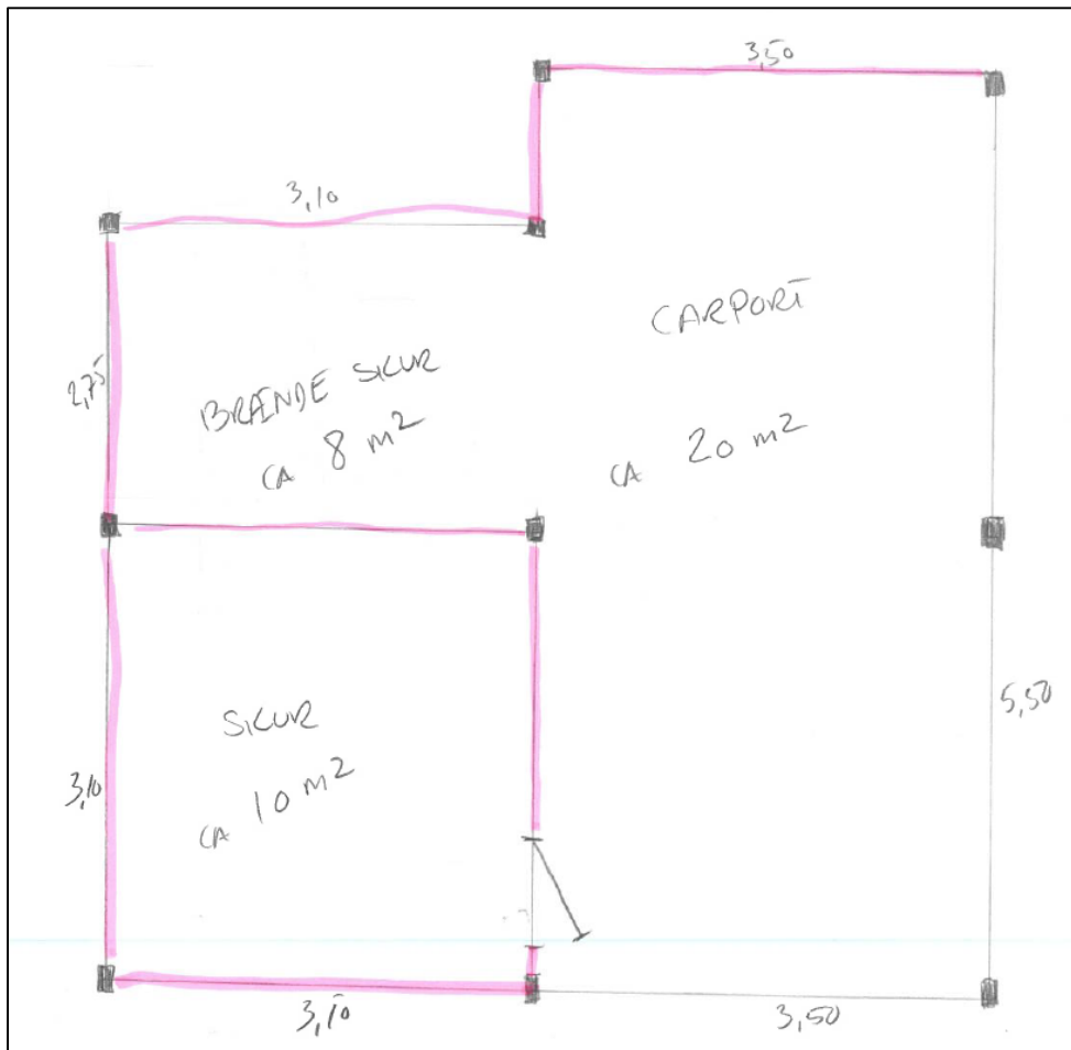
Tegning af det ansøgte indsat fra ansøgningen. Røde streger angiver lukkede sider. Højden på byggeriet er angivet til at være 2,3 meter. Indsat fra ansøgningen.
