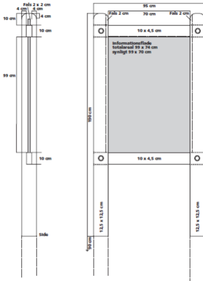
Fig. 4. Indsendt af ansøger. Illustrations af informationsskiltene med dimensioner. Bemærkning højde 1,8 m.
