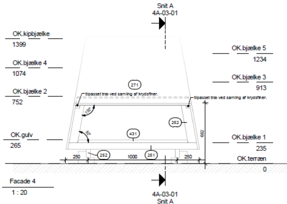
Facadetegning af shelteret Skrubben med mål.
