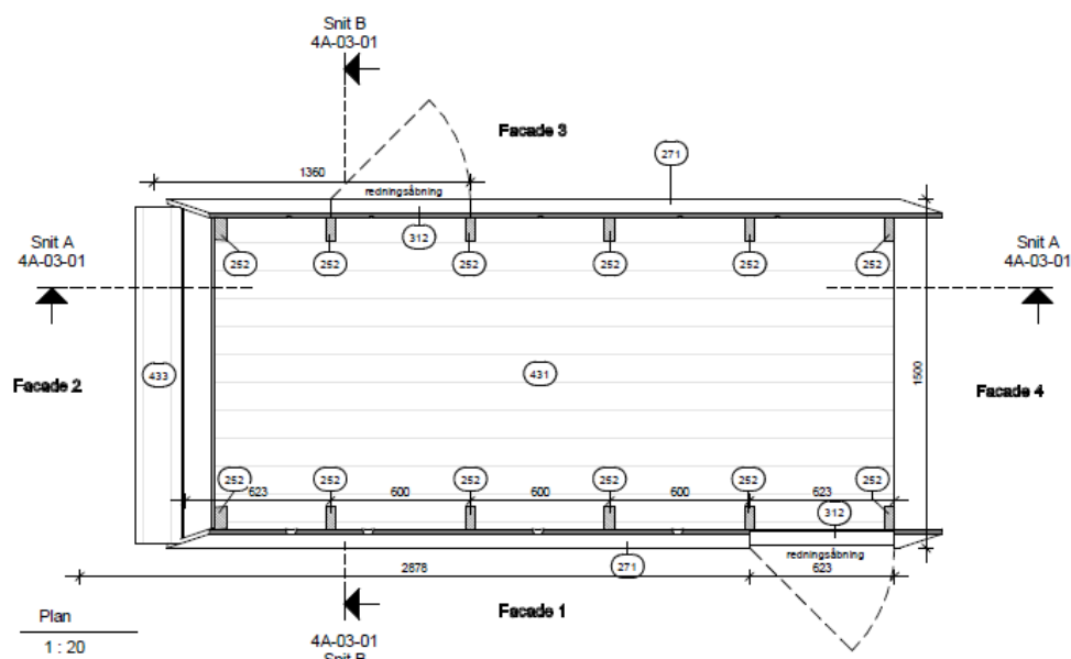
Plantegning af shelteret Skrubben med mål.
