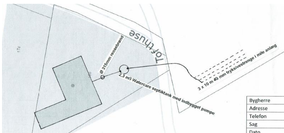
Kloakplan
