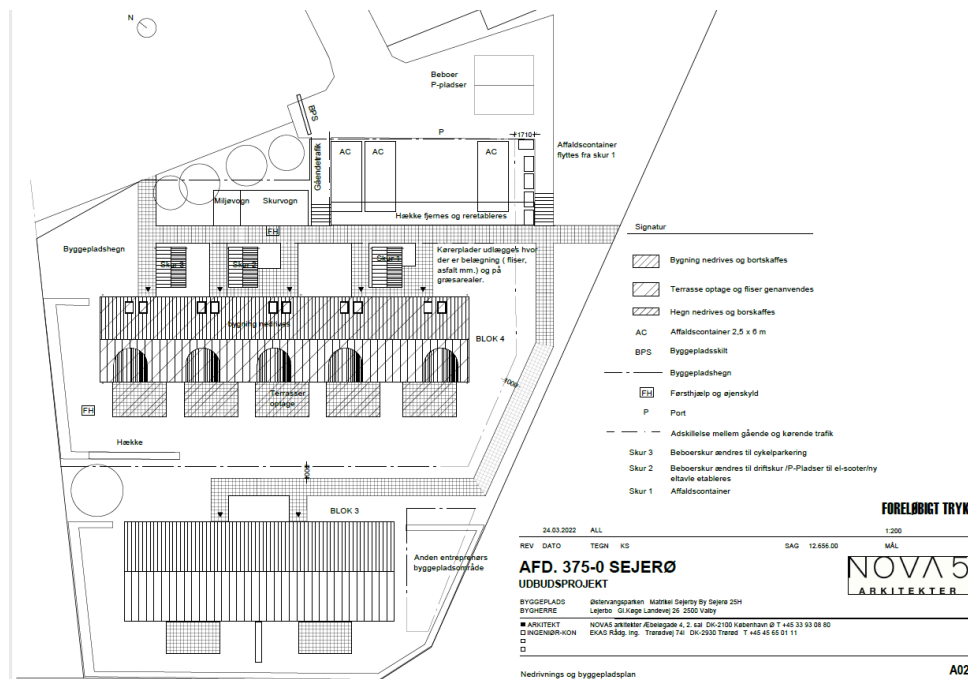
Hegning mv. af området ved nedrivningen – plan for arbejdsplads
