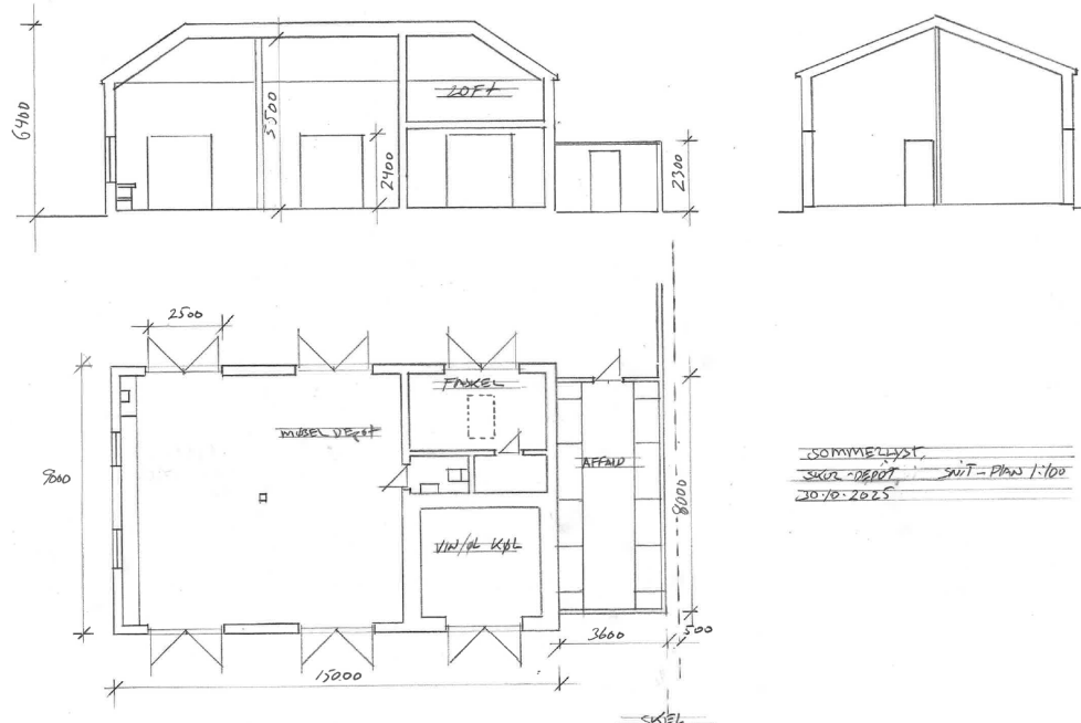
Fra ansøgningsmaterialet. Snit og plantegning af skur på arealet ved Ommelsvejen.
