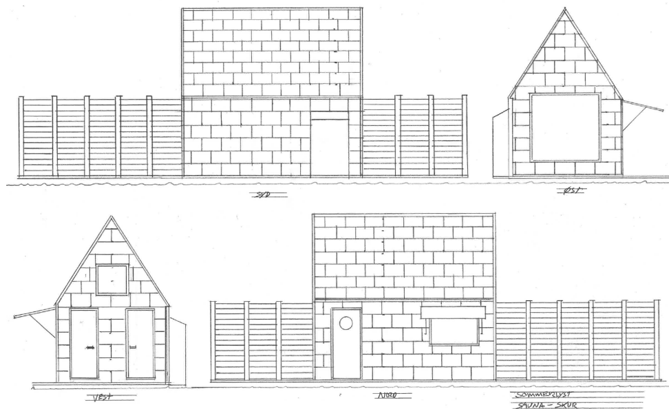
Fra ansøgningsmaterialet. Facadetegninger af sauna med depot og trædæk.
