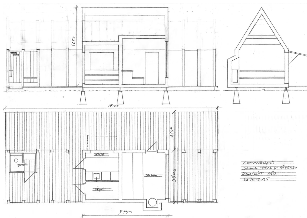
Fra ansøgningsmaterialet. Snit og plantegning af sauna med depot og trædæk.
