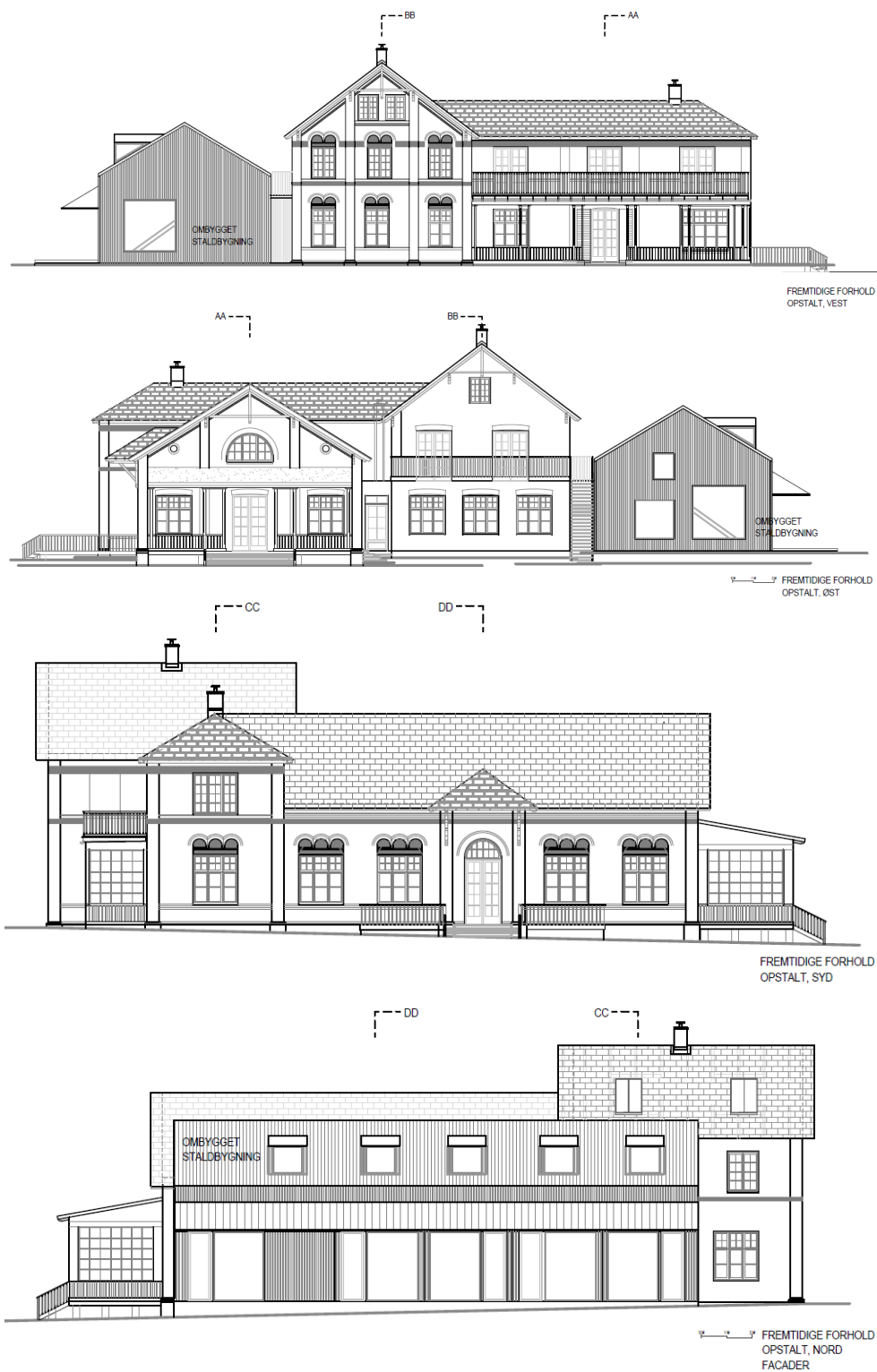
Fra ansøgningsmaterialet. Facadetegninger af fremtidige forhold.
