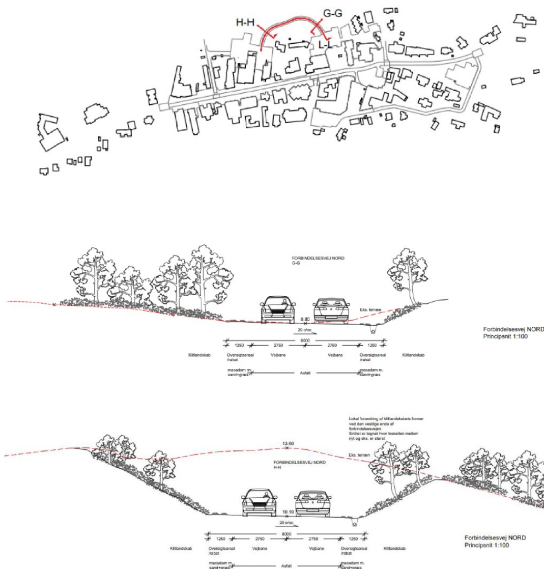
Figur 4. Skitser (tværsnit) fra ansøgningsmaterialet viser vejudlægget, herunder projekterede terrænenændringer.
