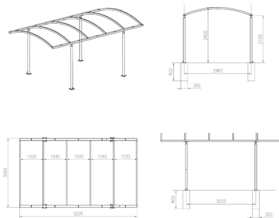
Fig. 5. Tilsendt fra ansøger. Tegning af ansøgte carport med mål.
