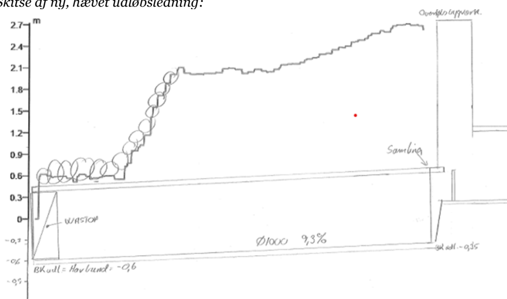
Skitse af ny, hævet udløbsledning:
