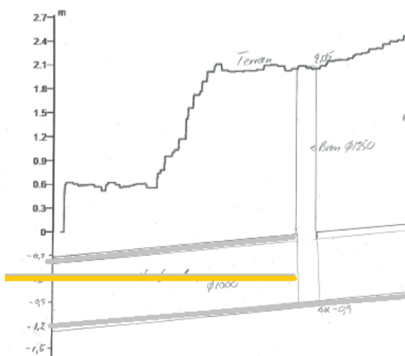
Skitse af eksisterende udløbsledning: gul (havbund) grå (ledningen)
