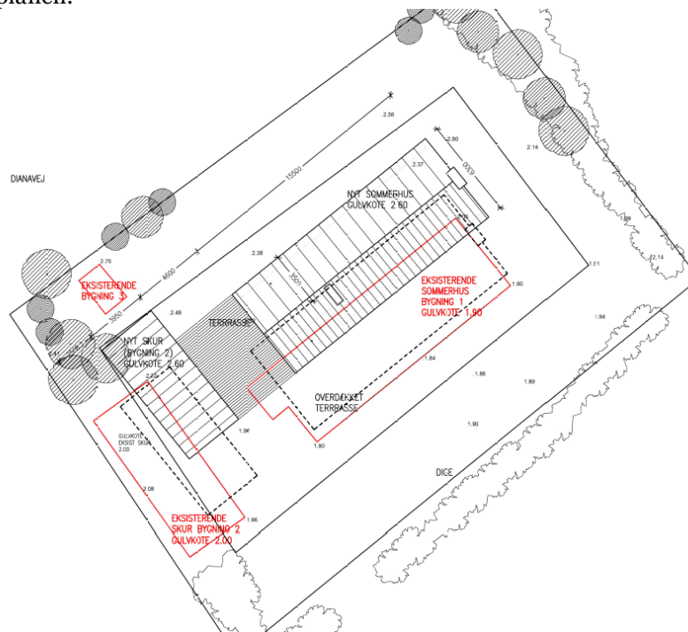
Situationsplan med ny placering af sommerhuset (stiplet gældende disp., og rød eksisterende hus)
