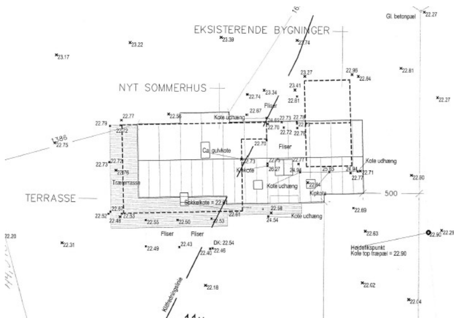
Figur 4: Situationsplanen for det fremtidige sommerhus. Det eksisterende er tegnet ind med stiplede linje
