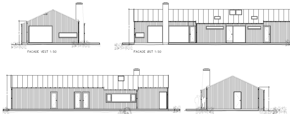
Figur 3: Tegningen af det fremtidige sommerhus
