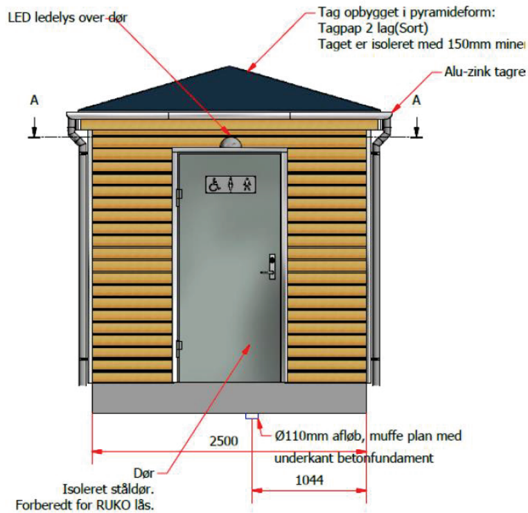
Fig. 3. Tilsendt fra ansøger. På figuren ses en principtegning af en toiletbygning.
