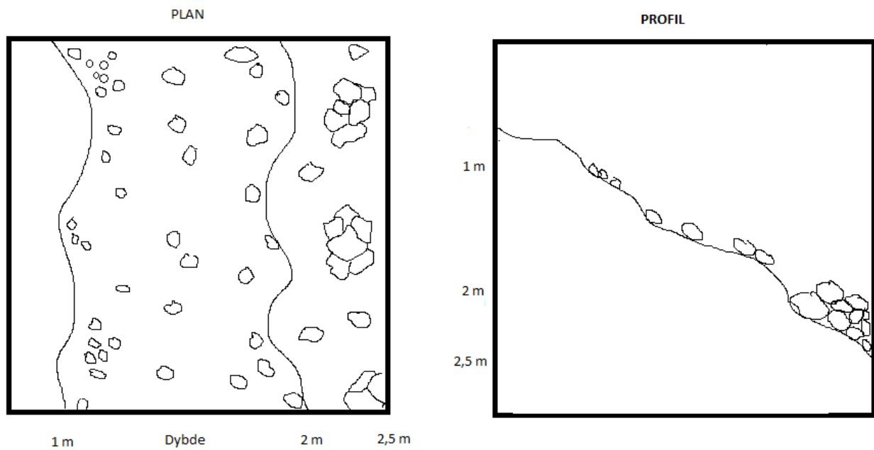
Figur 3: Skitse for udlægning af spredte sten. Til venstre er vist en planskitse og til højre en profilskitse. Af begge fremgår at stenene lægges ml. 1 m kurven og 2,5 m kurven.
