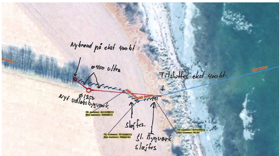
Situationsplan viser placering af nyt bygværk og rørføring.
