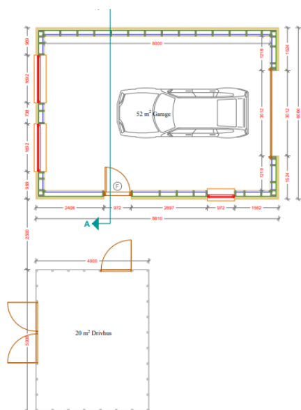
Grundplan garage og drivhus
