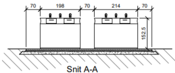
Fig. 4. Tilsendt fra ansøger. På figuren ses en plantegning af affaldsstation fra nord
