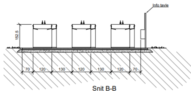
Fig. 5. Tilsendt fra ansøger. På figuren ses plantegning af affaldsstation fra øst
