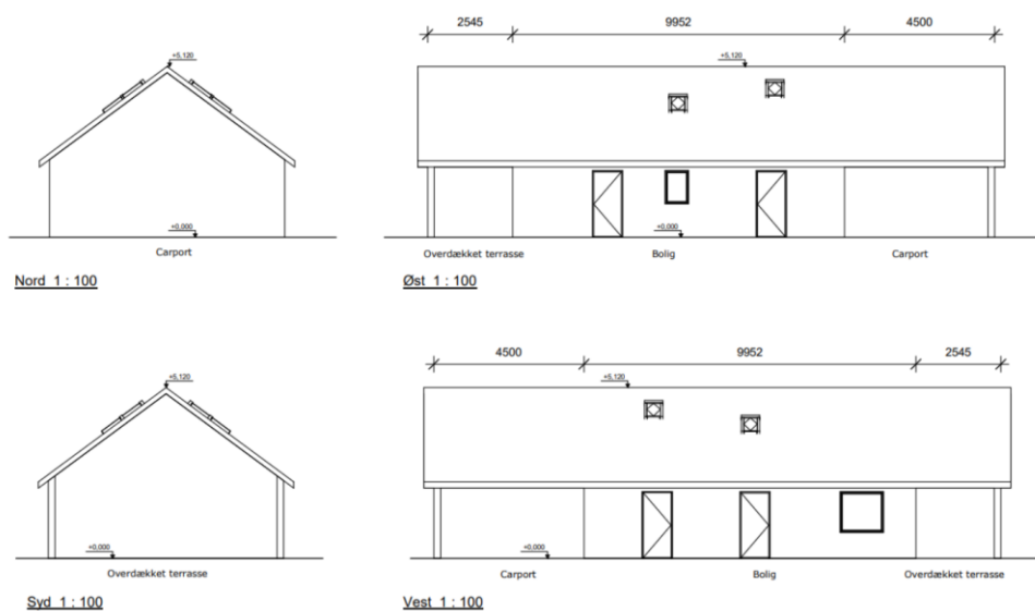
Fig. 4. Facadetegninger af ejendommens bolig indsendt af ansøger.
