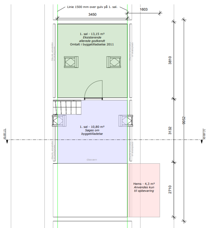
Fig. 2. Plantegning over boligens førstesal indsendt af ansøger. Som det fremgår af tegningen, markerer den grønne farve det eksisterende boligareal, mens den blå farve markerer den ansøgte udvidelse af boligarealet og lyserød/laksefarve markerer arealet, der ønskes anvendt til hems.
