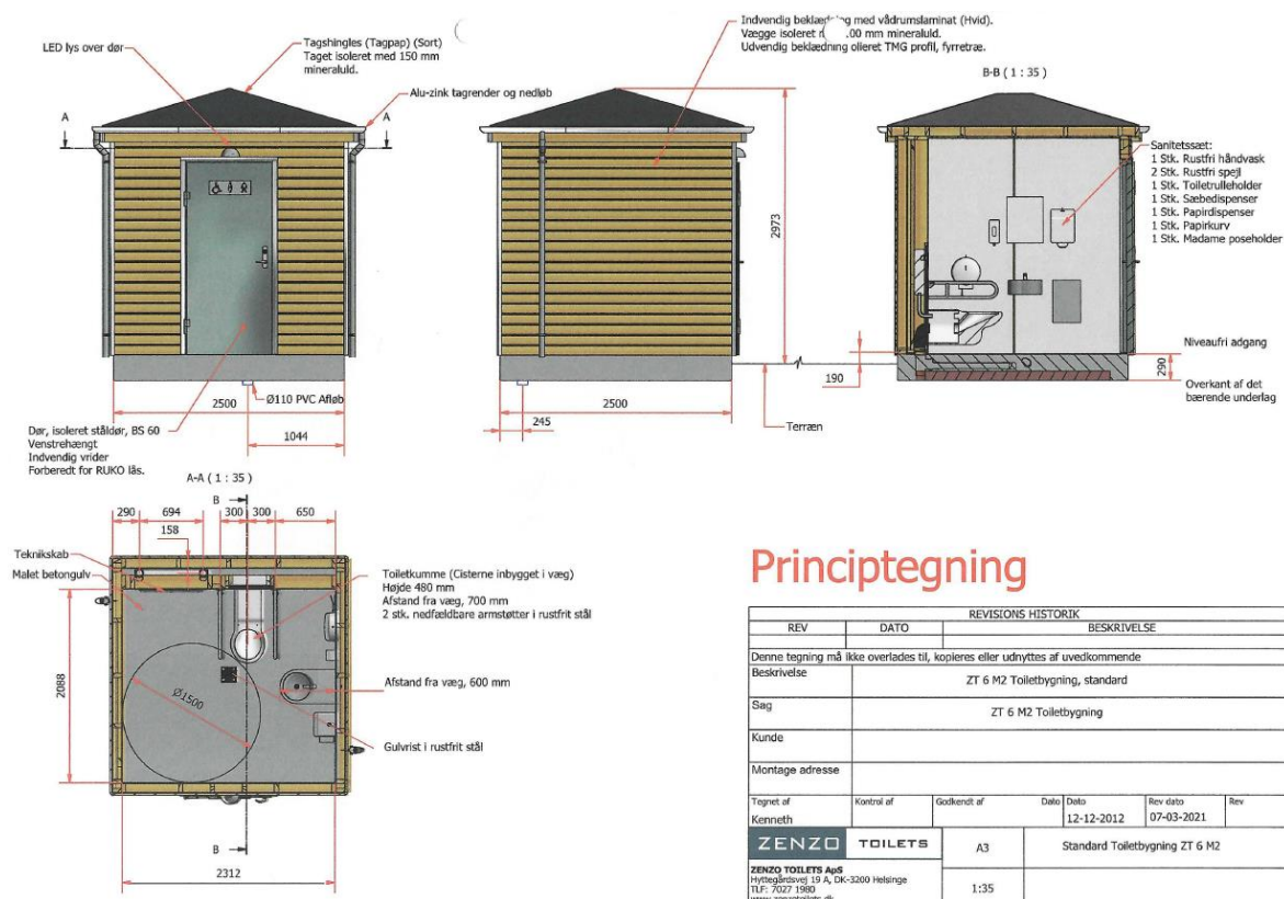
Fig. 4. Tilsendt fra ansøger. På figuren ses en principtegning over den ansøgte toiletbygning.
