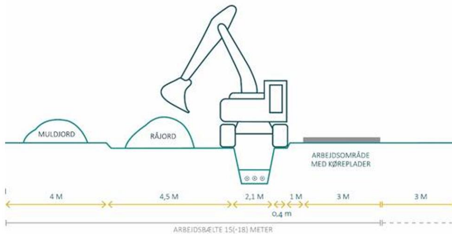
Princip for tværsnit af anlægsbælte
