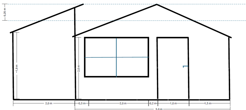
Skitse af forslag 2 til ændring af tagkonstruktionen.
