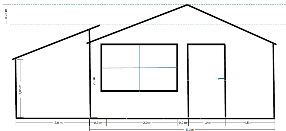
Snit af eksisterende forhold set fra syd. Sidebygningen til venstre.
