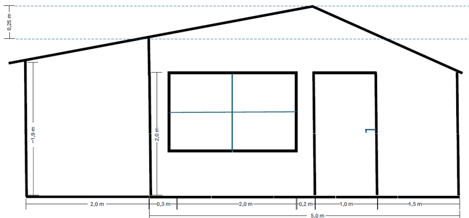
Skitse af forslag 1 til ændring af tagkonstruktionen
