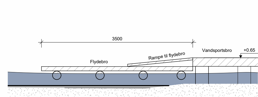
Snit - Flydebro 1 : 50
