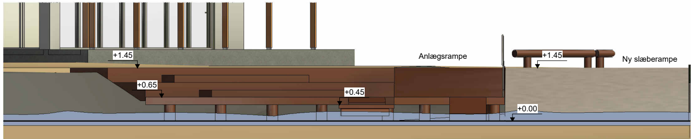
Opstalt - Vandsportsrampe 1 : 100
