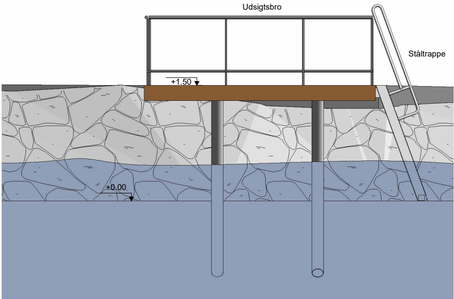
Opstalt - udsigtsbro set fra nord 1 : 50
