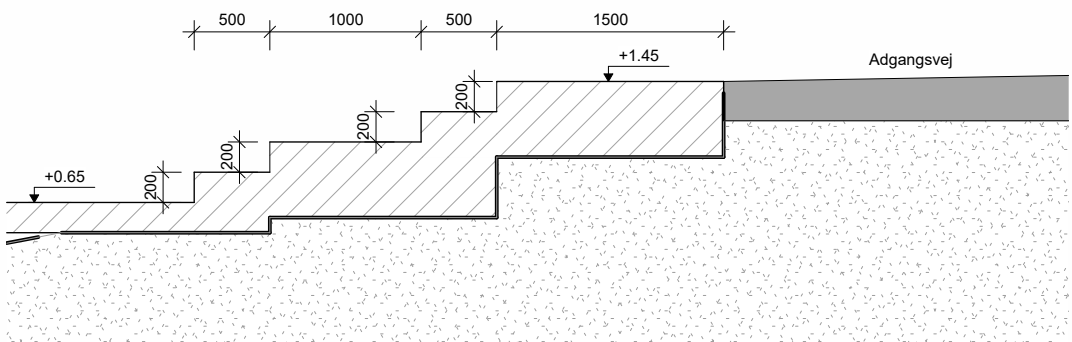
Snit - Trapper og siddepladser 1 : 50
