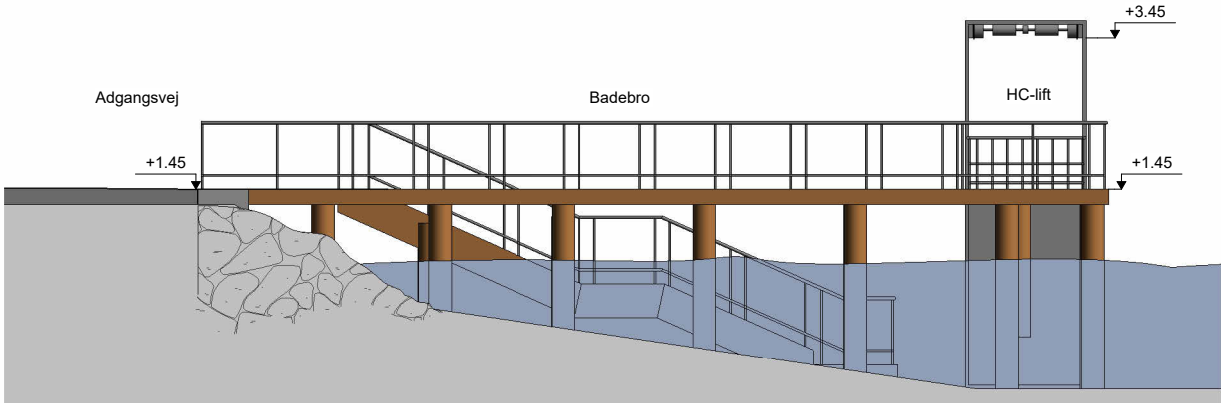
Opstalt - Badebro set fra nord 1 : 100
