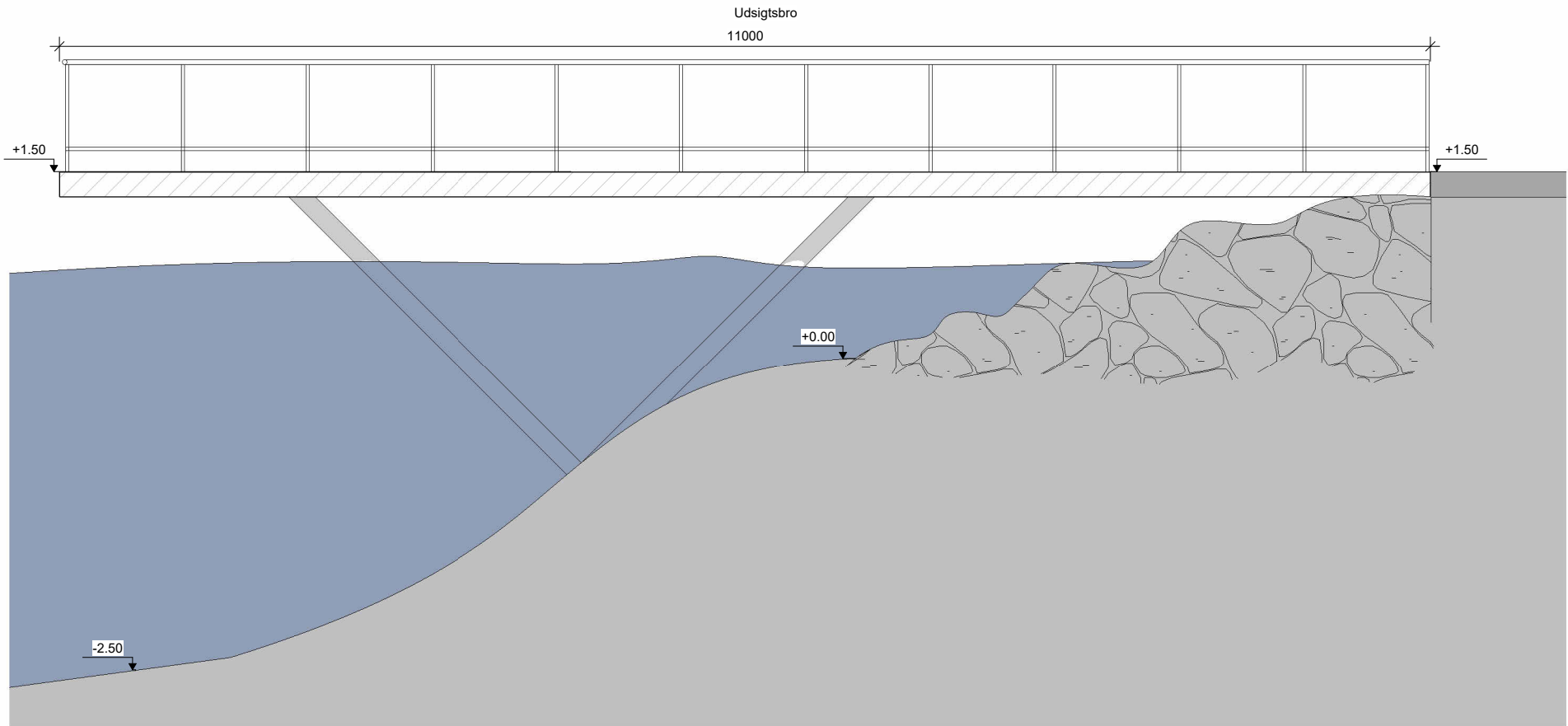
Snit udsigtsbro 1 : 50
