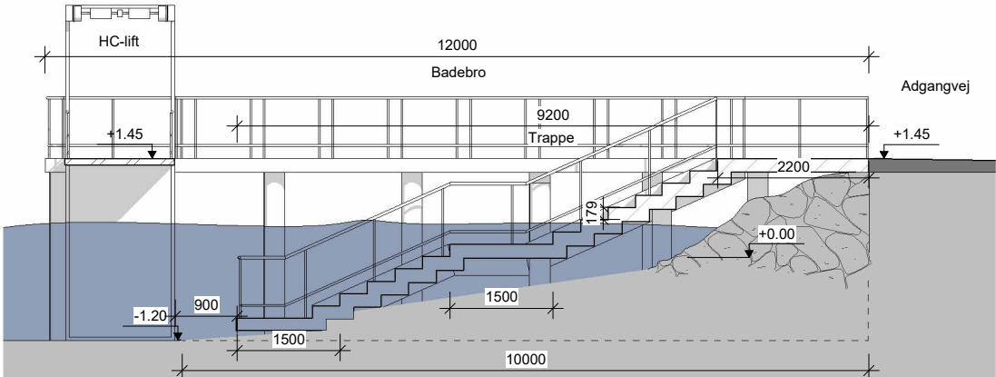
Snit - Trappe badebro 1 : 100
