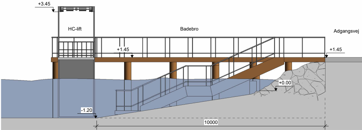
Opstalt - Badebro set fra syd 1 : 100
