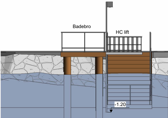
Opstalt - Badebro set fra vest 1 : 100
