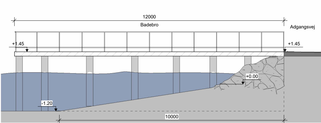
Snit - Badebro 1 : 100
