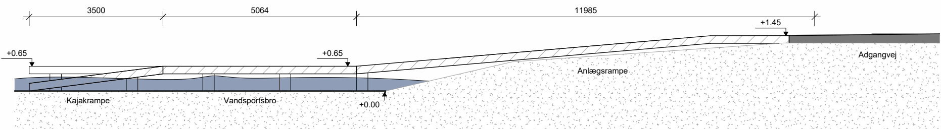
Snit - Vandsportsrampe 1 : 100
