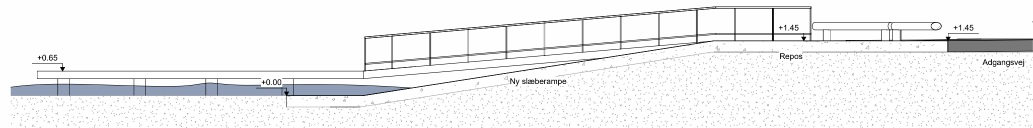
Snit - Slæberampe 1 : 100
