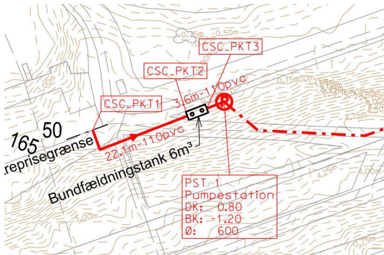
Figur 3 - Kloakanlæg ved Sdr. Pumpe
