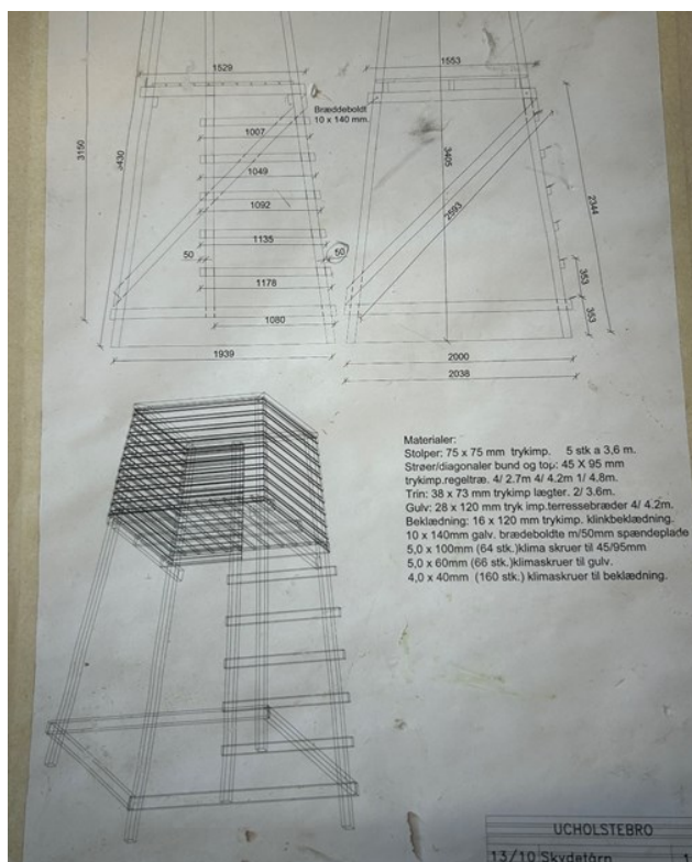
Tegning af skydetårnet med dimensioner
