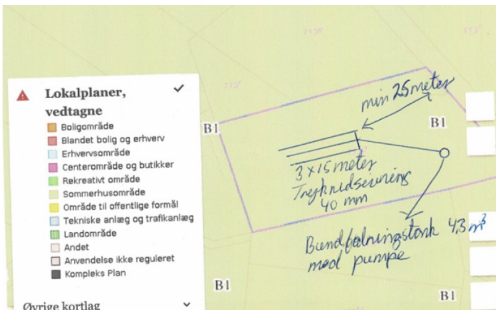
Situationsplan viser placering af bundfældningstank og sivedræn
