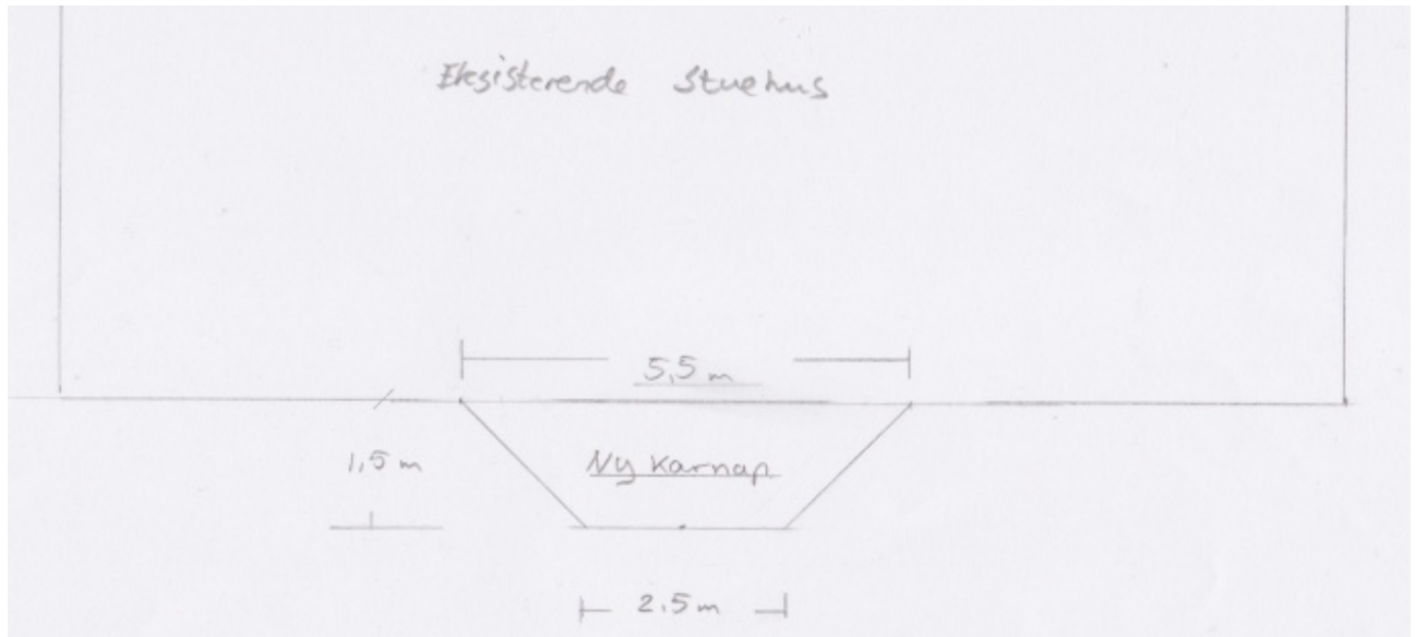
Fig. 8. Skitse af den påtænkte karnap med mål, indsendt af ansøger.
