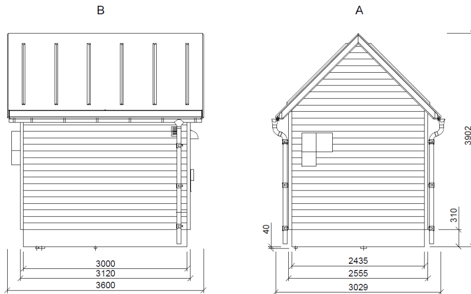
Fig. 3. Fremsendt billede til visuel illustration af toiletbygning.
