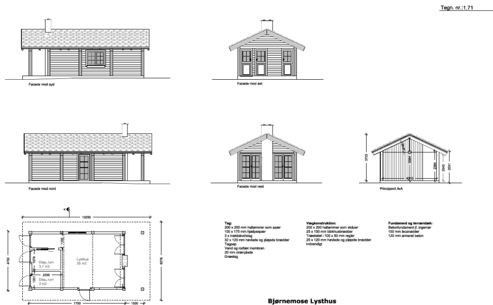
Figur 3, plan, snit og facadetegninger fra ansøgning
