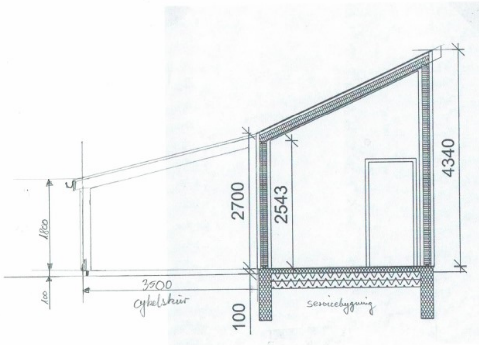
TVÆRSNIT CYKELSKUR - SERVICEBYGNING V. VENØ FÆRGEN SØNDERSKOVVEJ 26, VENØ
