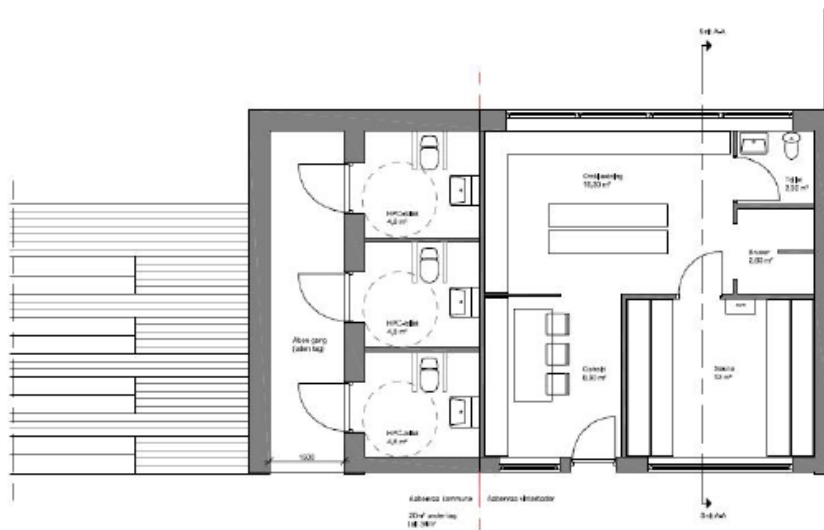
Plantegning
