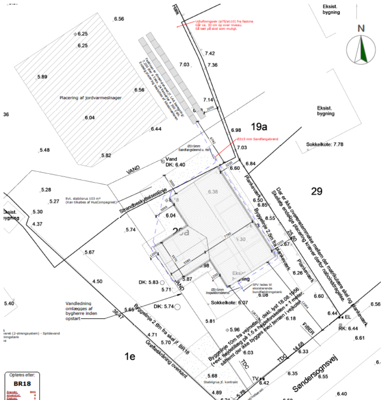
Fig. 2. Tilsendt fra ansøger: byggeplan for matriklen med strandbeskyttelseslinjen. Midlertidige terrænændringer er tegnet ind, synlige anlæg er markeret med rød skrift hhv. dæksel til sandfangsbrønd og udluftningsrør til faskine.
