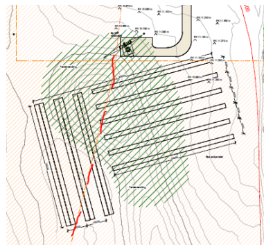
Grøn skravering område der terrænreguleres
