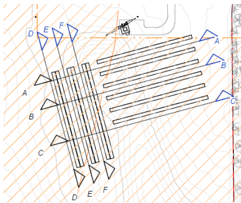
Snit B-B og F-F vist neden for
