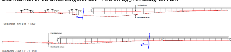
Snit B-B og F-F vist neden for
