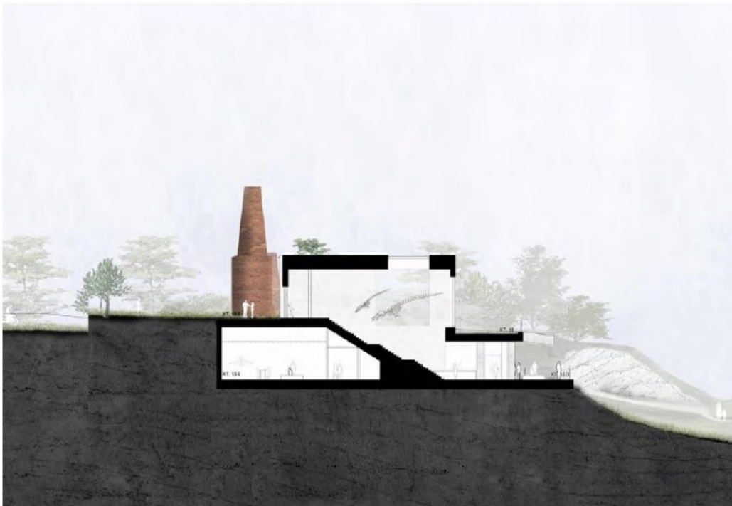
Fig. 5. Tværsnit af besøgscenter fra Lokalplan 200.
