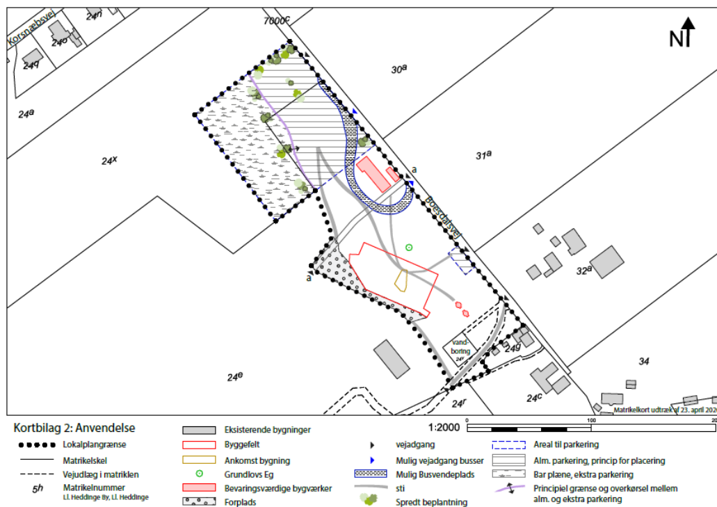
Fig. 3. Kortbilag 2 fra Lokalplan 200 med anvendelse af arealet, hvor byggefeltet for besøgscenteret mm. fremgår.
