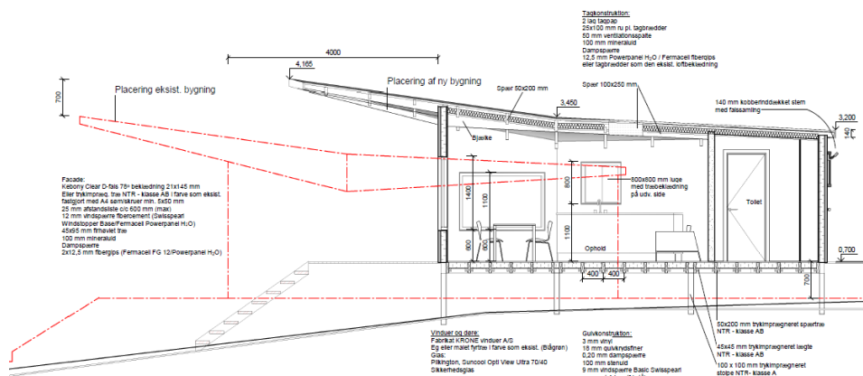
Tegning af eksisterende og nyt badehus. Eksisterende med rød stiplede strek.
