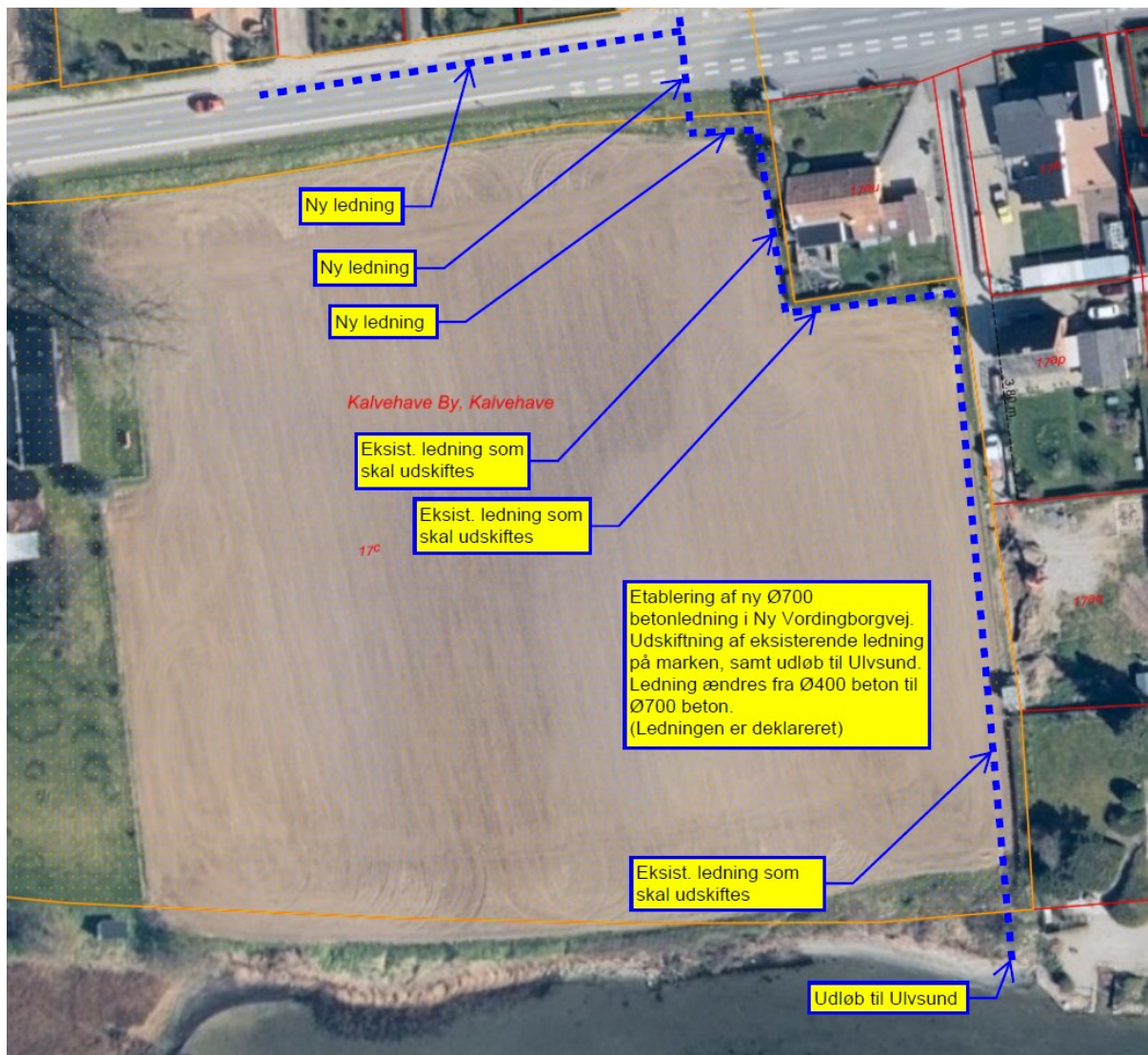
Forløb af ny ledning og ledning, som udskiftes.
