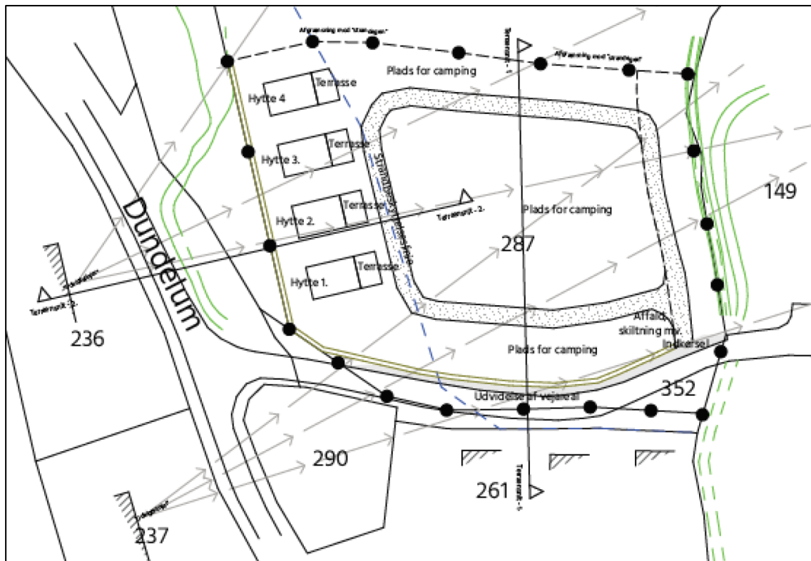
Situationsplan for udvidelsen. Strandbeskyttelseslinjen er vist med blå stiplede linje. Hytter opføres uden for det strandbeskyttede areal.
