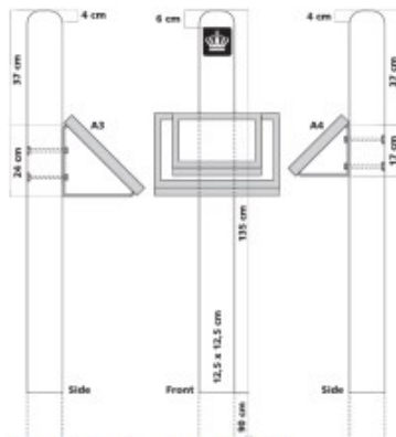
Figur 5 - infotavler, dimensioner, A3
