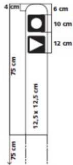
Figur 3 - Rutepæl, dimensioner
